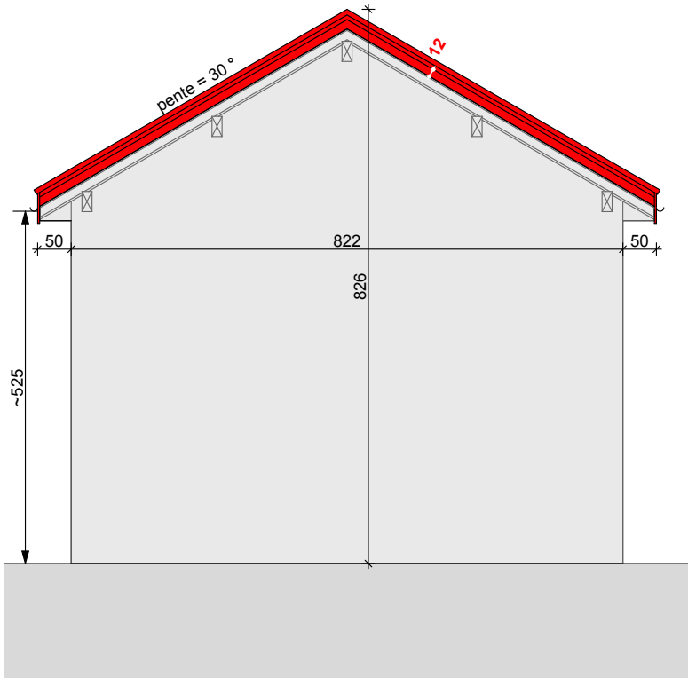
COUPE TOITURE 1:100 (MAISON EXISTANTE)
