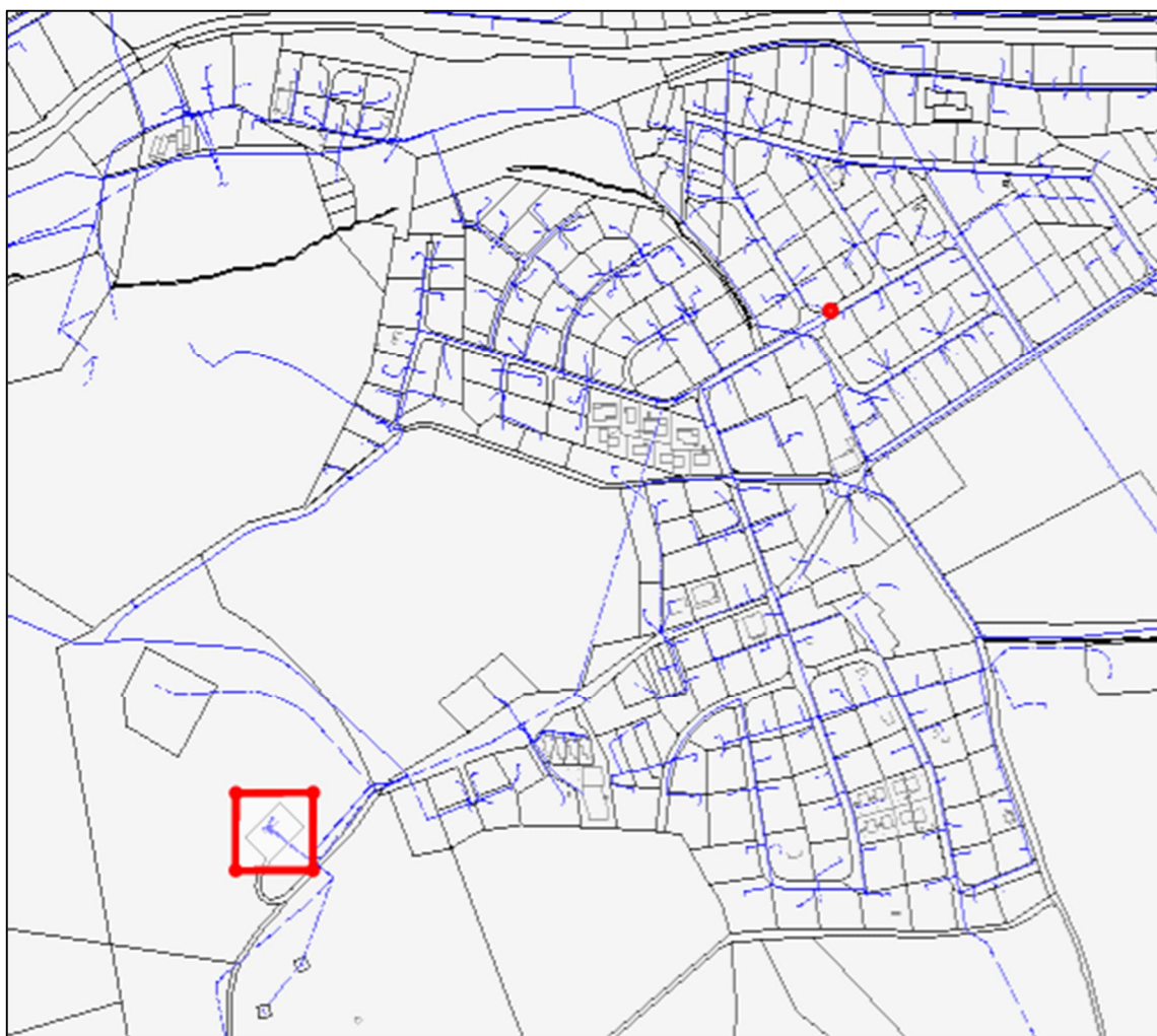
Réservoir des Borcards (carré rouge) et chambre de vanne (point rouge)
